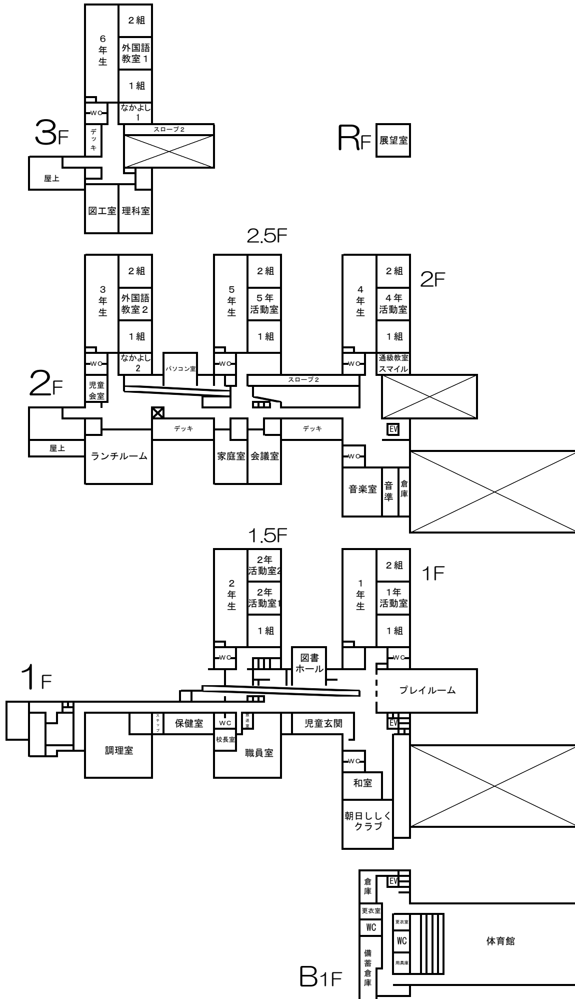
【校舎平面図】
