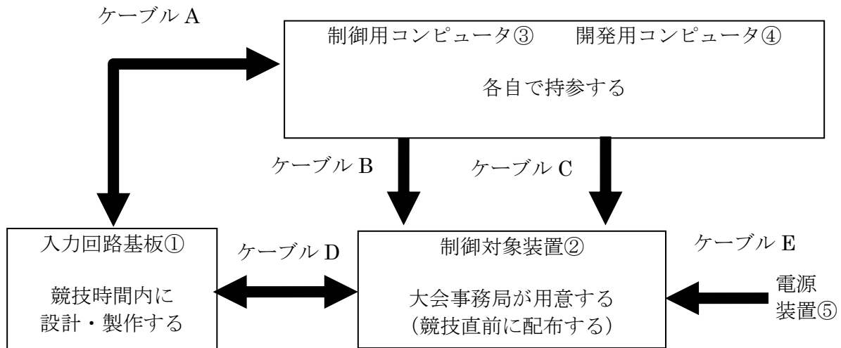
図 1 課題システムの構成図
