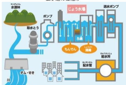
上水道の仕組み
